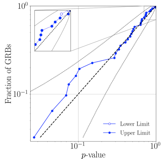
Rysunek 1: W metodzie poszukiwania fal grawitacyjnych przy użyciu modelu brany pod uwagę jest najlepszy kandydat dla każdego krótkiego GRB wraz z pomiarem jego wiarygodności statystycznej. Porównujemy to z danymi dla innych przedziałów czasowych, aby oszacować prawdopodobieństwo, że kandydat jest wynikiem szumu, a nie fali grawitacyjnej ( wartość p ). Na wykresie przedstawione są wyniki dla 32 kandydatów (połączone kropki), przy czym oś pozioma daje wartości wartości p , a oś pionowa pokazuje ułamek kandydatów, z niższą wartością p . Linia przerywana jest krzywą, jakiej można by się spodziewać po samym szumie detektora tła i przypadkowej szansie detekcji (i braku fal grawitacyjnych). Im większa jest wartość p (dalej w prawo), tym większa jest szansa, że jest to zdarzenie jest szumem, a nie falą. Liniami kropkowymi zaznaczono granice oczekiwanego statystycznego zachowania się szumu w naszych poszukiwaniach. Widzimy, że wszyscy kandydaci (połączone kropki) znajdują się w obrębie linii kropkowych, co oznacza, że wszystkie są zgodne z tym, czego można oczekiwać od tła szumu detektora.
