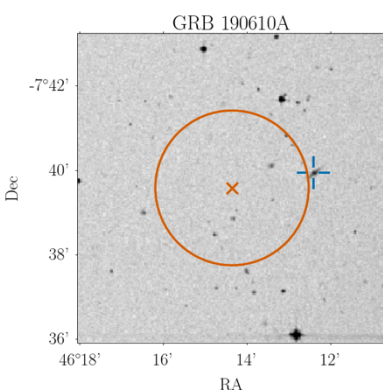
Rysunek 5: Okrąg na wykresie oznacza zakres błędów pozycji dla GRB190610A, błysku który mógł wystąpić w galaktyce odległej od nas o około 165 Mpc (około 600 milionów lat świetlnych stąd), zaznaczonej niebieskim krzyżem. Odległość ta jest większa niż „odległość wykluczenia” (Rys. 3 i 4) dla tego GRB, więc być może blysk powstał w tej galaktyce, ale znajduje się ona zbyt daleko, by nasze detektory wykryły fale grawitacyjne.
